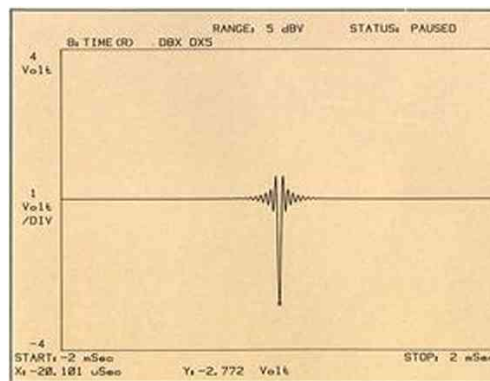
Impulsresponsen är symmetrisk vilket ger en rak fasgång.
