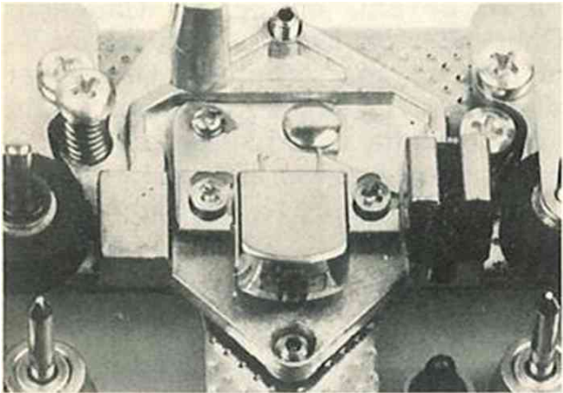
SPECIALTONHUVUD av "supcr-permalloy"-typ utvecklat av I and berg.
