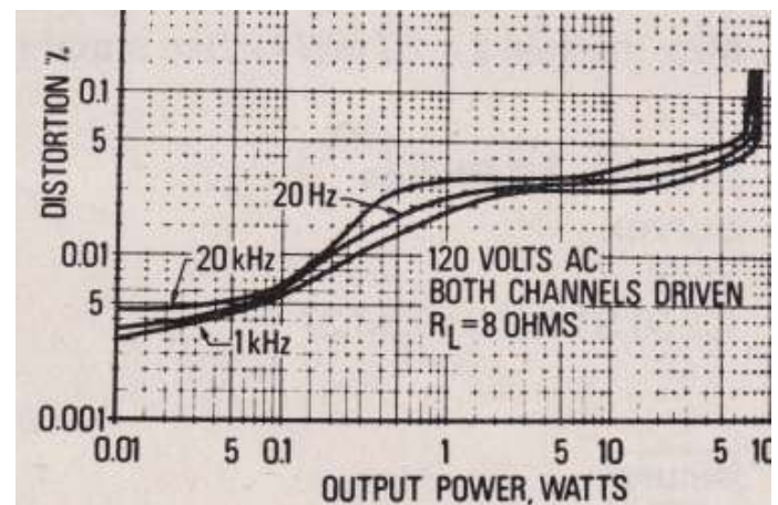
Distorsion som funktion av uteffekten (båda kanalerna drivna).
