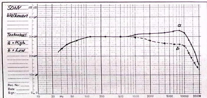
Frekvenskurva med tonkontrollen i läge High (a) och läge Low (b).
