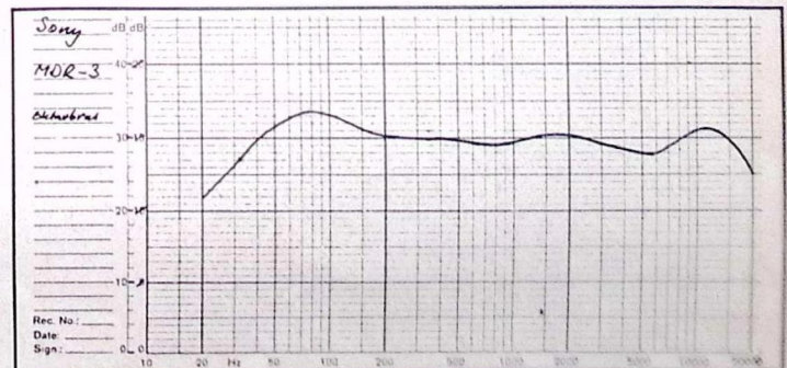
Frekvenskurva för Sony hörtelefon MDR-3 mätt med brus som signal och mätmikrofon i stället för örat.
