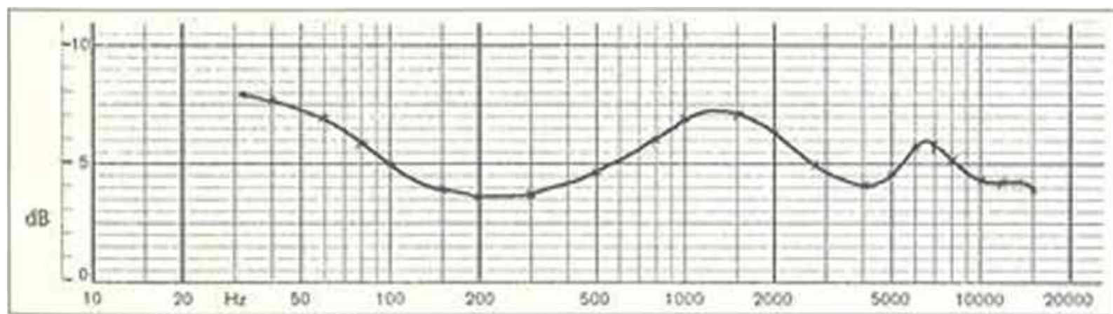
Frekvenskurva för Pioneer SE-M10
