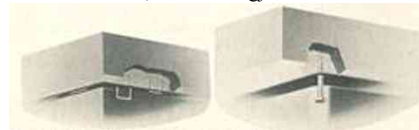
VANLIGA HÄFTKLAMRAR LOSSNAR LÄTT. DÄRFÖR HAR PIONEER FÖRSEGLAT BASPLATTAN I LÅDAN MED ALUMINIUMSKRUVAR.
