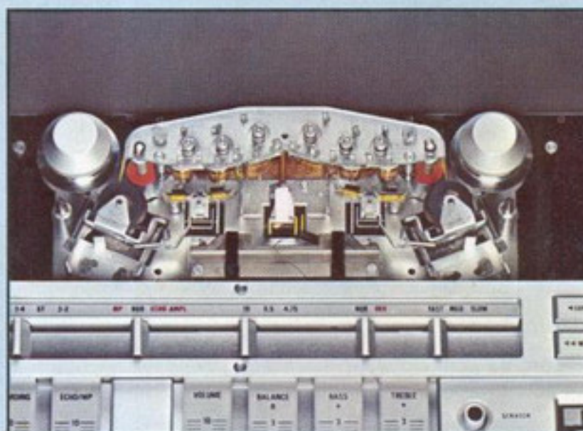
6 Tonköpfe und 2 Tonwellen. Darunter Bandklebeschiene.
