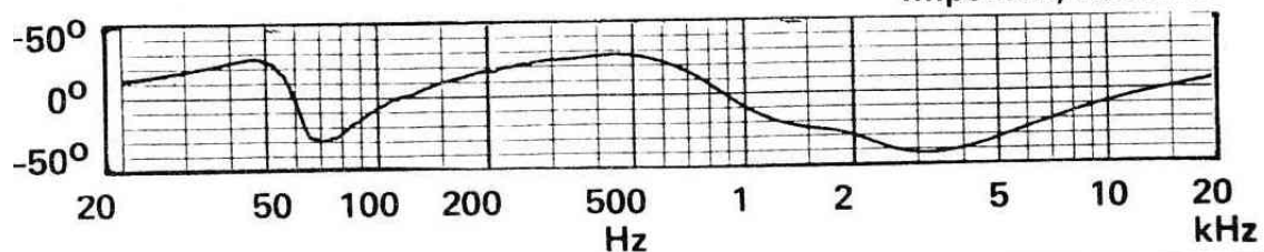
Impedans, fasvinkel
