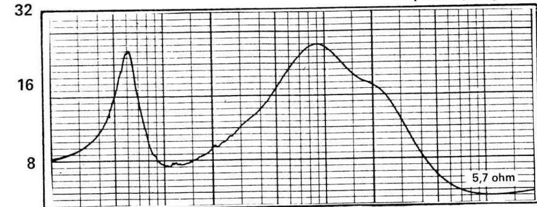
Impedans, fasvinkel
