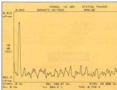
Spelaren har ett lågt kvantiseringsbrus.
