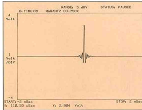
Impulsen är helt symmetrisk vilket ger en rak fassgång.
