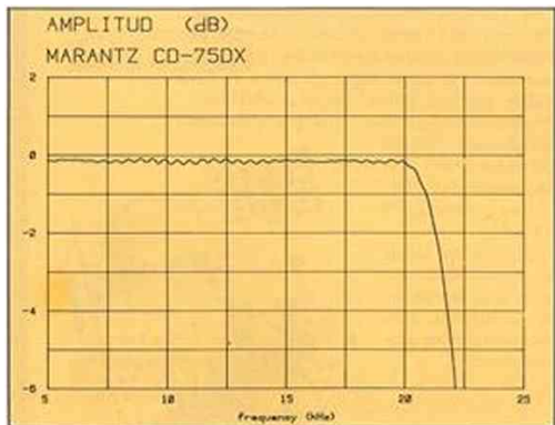
Amplitudkurvan har ett mycket rakt förlopp.
