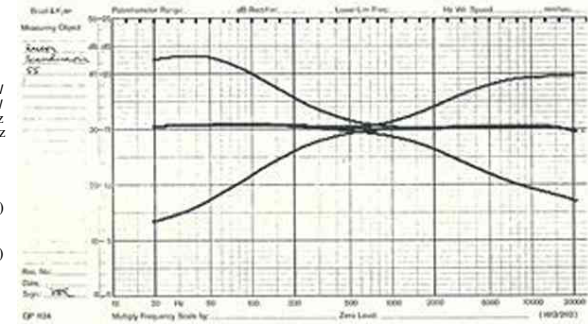
Frekvensgång med tonkontroller i min., mitt- och max-lågen, se kurva t.v.
