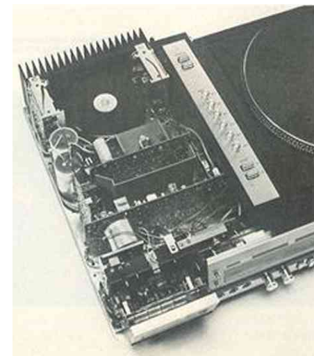
I apparatens vänstra del sitter det mesta av elektroniken. Framst ser man bandspelaren och bak till närttransformatorn av ringkärntyp samt de båda effektförstärkarna med kylflänsar.
