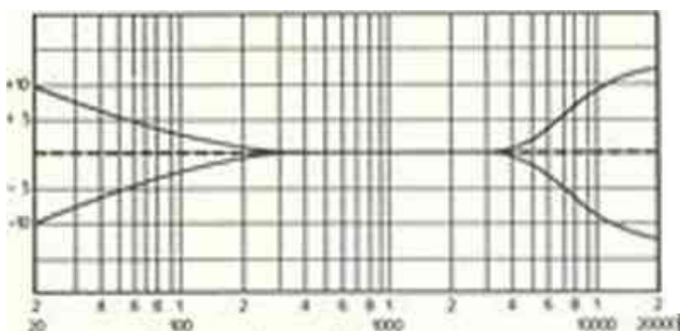
Konventionell tonreglering
